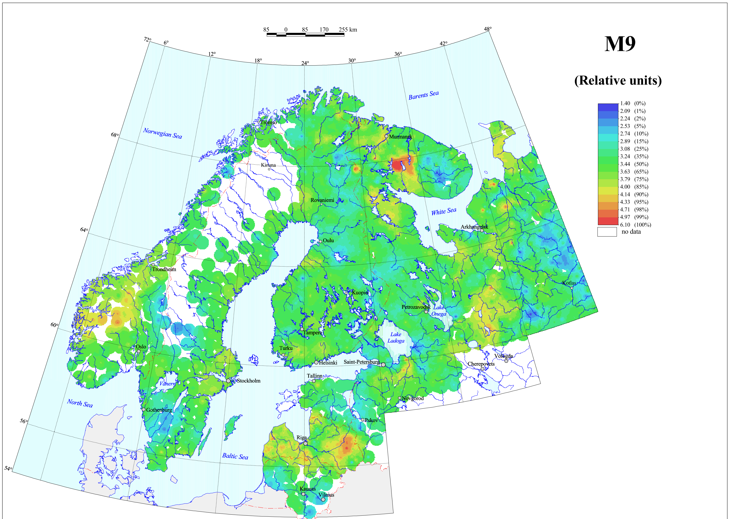
M9 (P, Sr) in C-horizon, Grain Size <2 mm, Aqua regia Extraction
